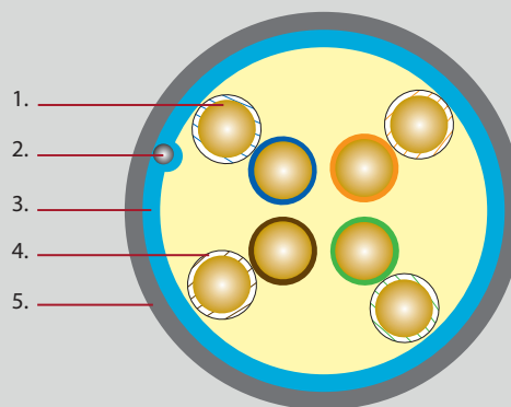
DIXON 8040 4P x 24 AWG – STP CAT5E
