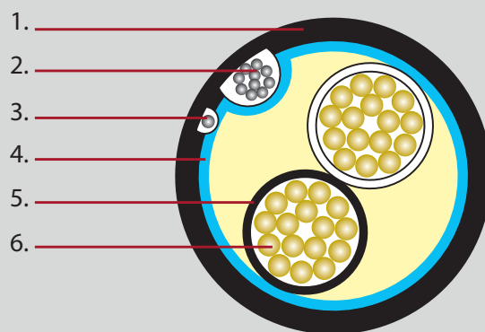
Dixon 8010 LSZH 2C x 18 AWG
