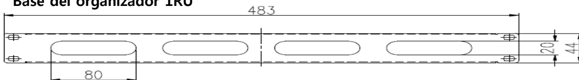
Base del organizador 1RU
